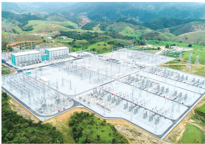
这是位于巴西里约热内卢州的美丽山水电站二期输电项目里约换流站（2019 年 11 月 6 日摄）。美丽山水电站二期输电项目由中国国家电网独立中标，将巴西北部的清洁水电输送至东南部，为巴西打造一条“电力高速公路”。 新华社发（国家电网巴西控股公司供图）
