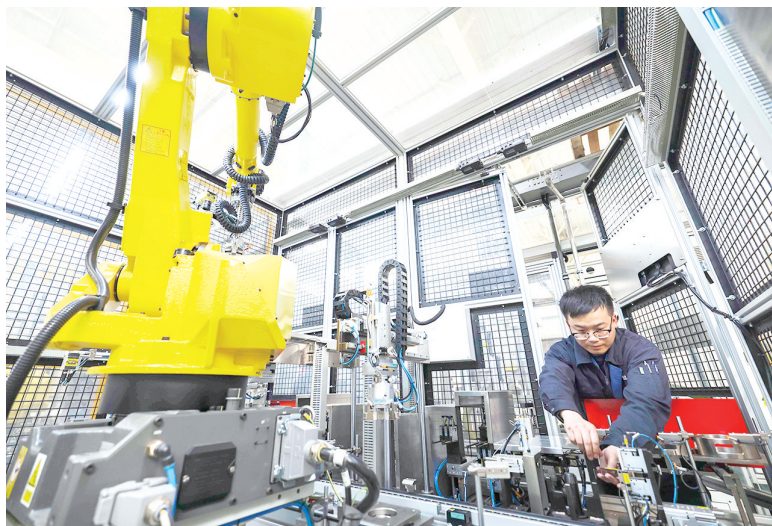
4月27日，工人在位于江苏省泰州市姜堰区的江苏太平洋精锻科技股份有限公司生产车间忙碌。 新华社发
